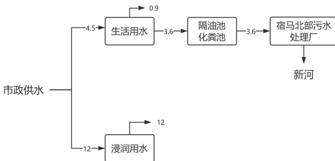
图 2-1 本项目建成后水平衡图 单位: t/d
