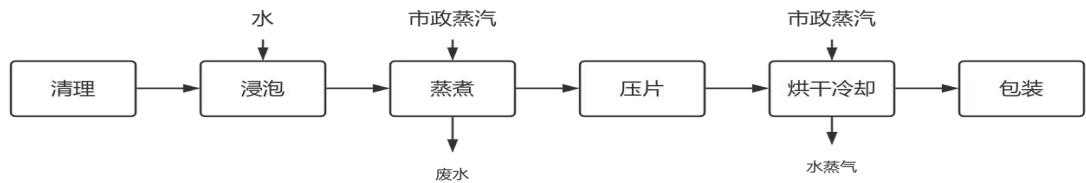
图 2-2 玉米压片工艺流程图
