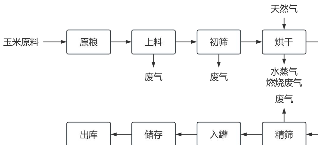
图 2-1 玉米原粮处理工艺流程
