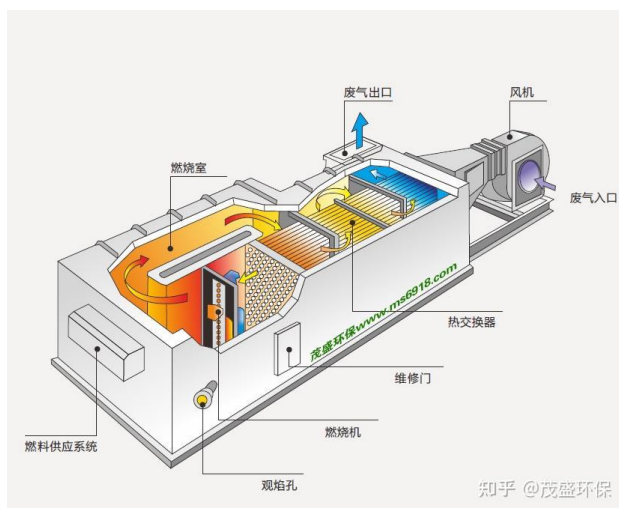
图 4-1 TO 直燃烧炉结构示意图
