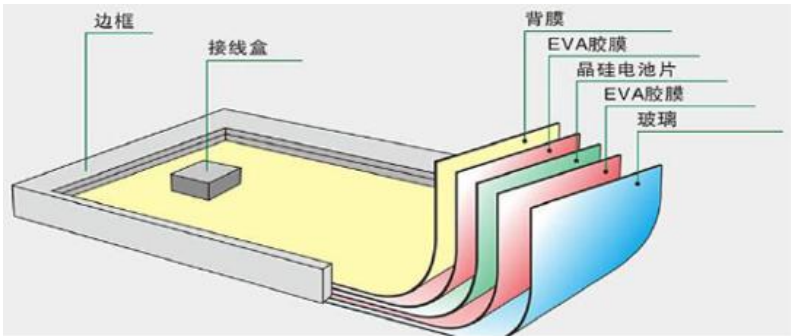
图 2-1 单玻晶硅光伏组件结构示意图
