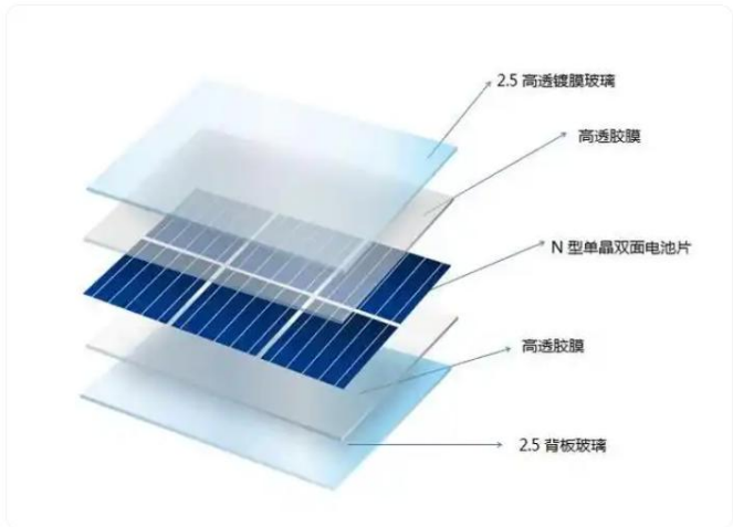
图 2-2 双玻晶硅光伏组件结构示意图
