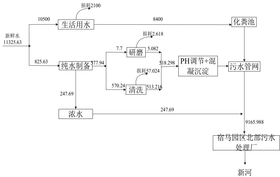
图2-1 项目水平衡示意图 单位：t/a
